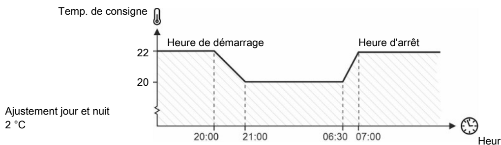
Figure 8: Le réglage jour et nuit est défini comme un abaissement nocturne de la température.
