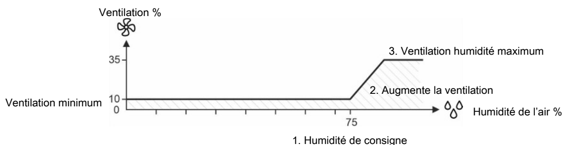
Figure 11: Ventilation de l'humidité : 1. L'humidité de l'air dépasse le point de consigne d'humidité. 2. Le contrôleur augmente la ventilation. 3. Augmentation jusqu'à la ventilation maximale d'humidité (35 %).
