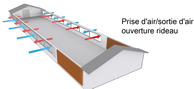
Figure 18: Exemple de bâtiment d'élevage avec la ventilation naturelle en association avec la ventilation tunnel, Ventilation naturelle.
