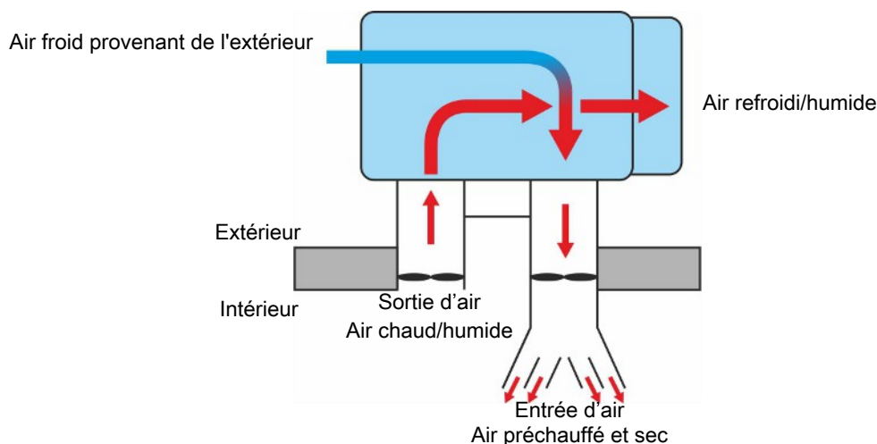
Figure 14: Exemple du principe de l'unité de récupération de chaleur.
