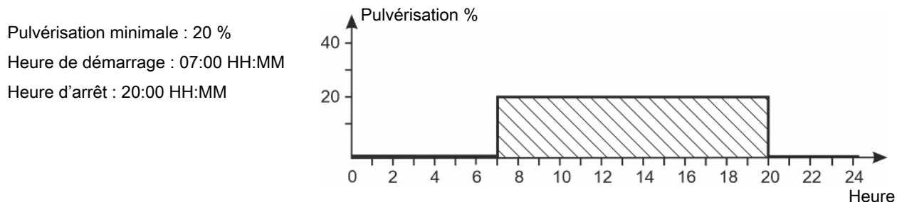
Figure 29: Pulvérisation conformément à l'heure
