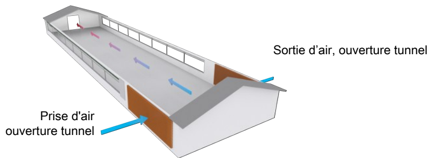
Figure 19: Exemple de bâtiment d'élevage à ventilation naturelle combiné à une ventilation tunnel, Ventilation tunnel.
