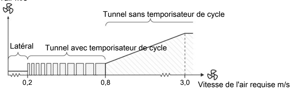
Figure 16: Séquence de ventilation avec temporisateur de cycle en ventilation mode tunnel
