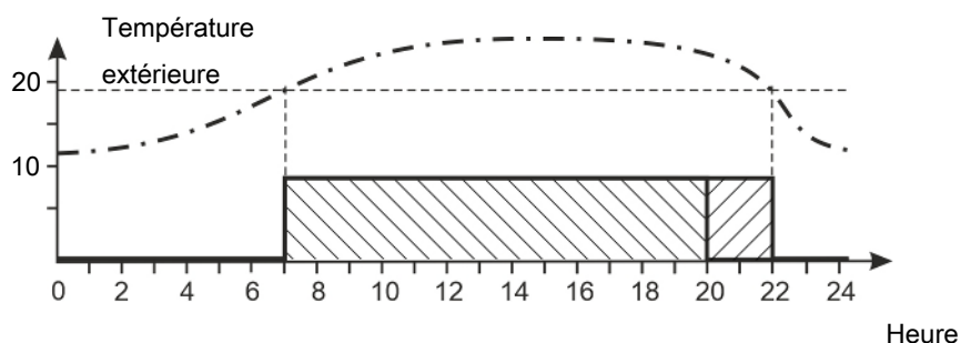
Figure 30: Pulvérisation conformément à l'heure et à la température extérieure
