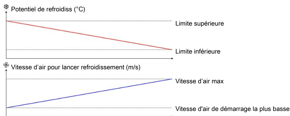
Figure 31: Dans les zones à faible humidité extérieure et à fort potentiel de refroidissement, le refroidissement peut démarrer à une vitesse d'air plus faible. Dans les zones à faible potentiel de refroidissement, le refroidissement démarre le plus tard possible, ce qui signifie qu'il démarre à une vitesse d'air maximum.
