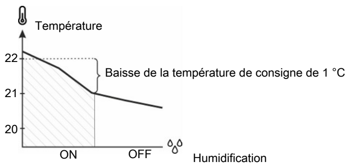
Figure 10: Diminution de la température : L'humidification sera déconnectée si la température intérieure est inférieure de 1 °C à la Température de consigne. Autrement, l'humidification peut faire chuter davantage la température intérieure.
