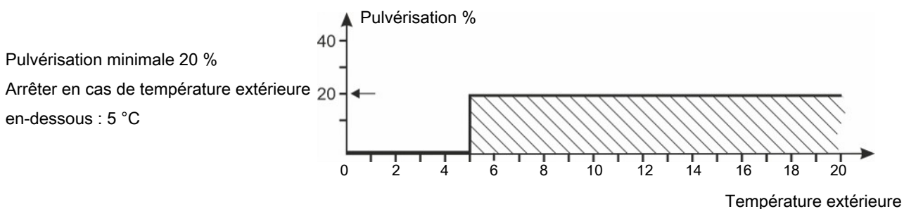
Figure 28: Pulvérisation conformément à la température extérieure
