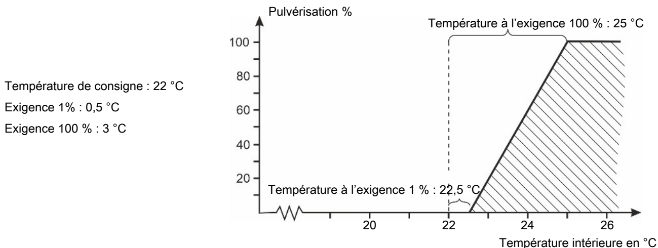
Figure 27: Pulvérisation conformément à la température intérieure
