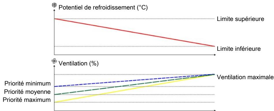
Figure 26: Plus le potentiel de refroidissement est élevé, plus la priorité de démarrage anticipé du refroidissement est élevée.
