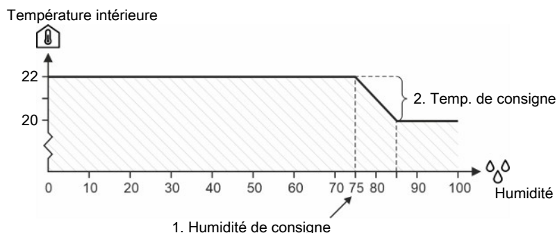
Figure 12: Contrôle de l'humidité avec réduction de température
