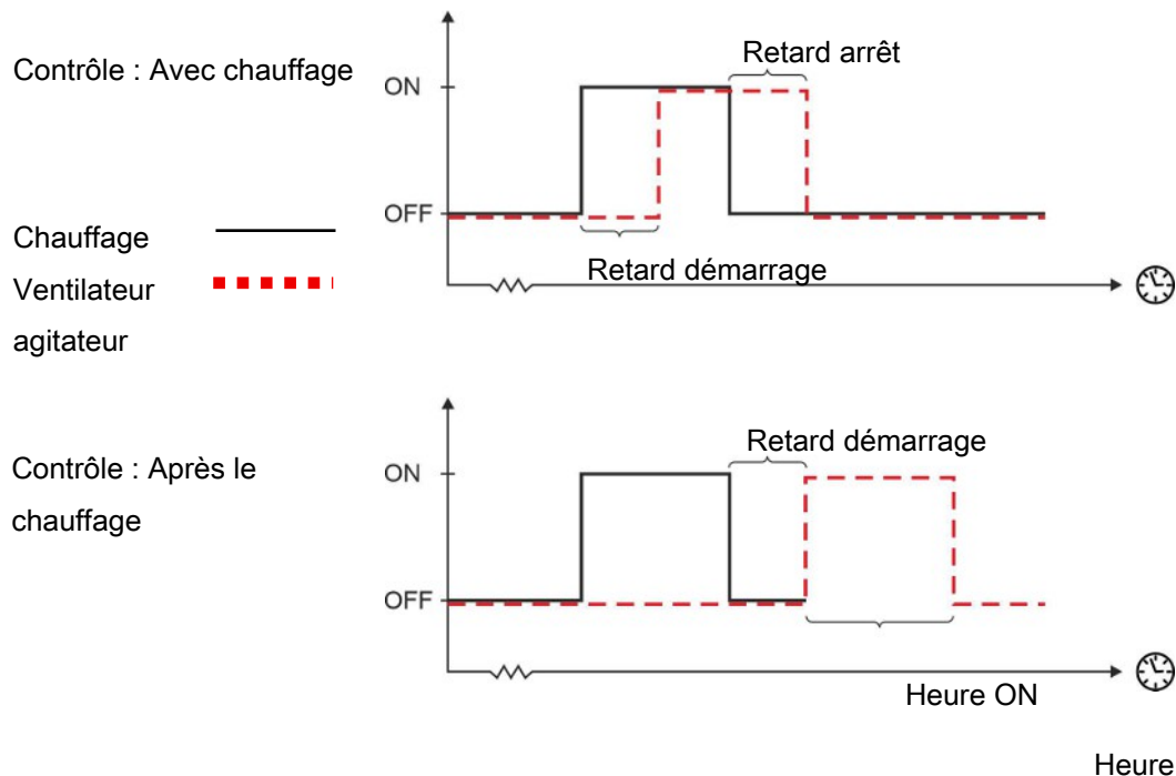
Figure 23: Contrôle avec chauffage
