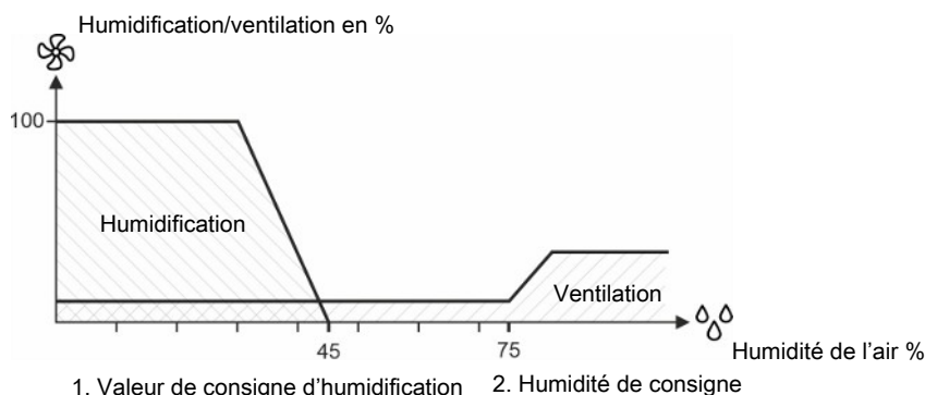
Figure 9: 1. Diminution de l'humidité de l'air. L'humidité de l'air est inférieure au point de consigne d'humidification. Le contrôleur démarre l'humidification. 2. Augmentation de l'humidité de l'air L'humidité de l'air est supérieure au point de consigne d'humidité. Le contrôleur augmente la ventilation.
