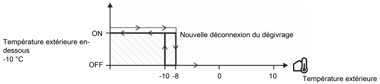
Figure 13: Activation du dégivrage
