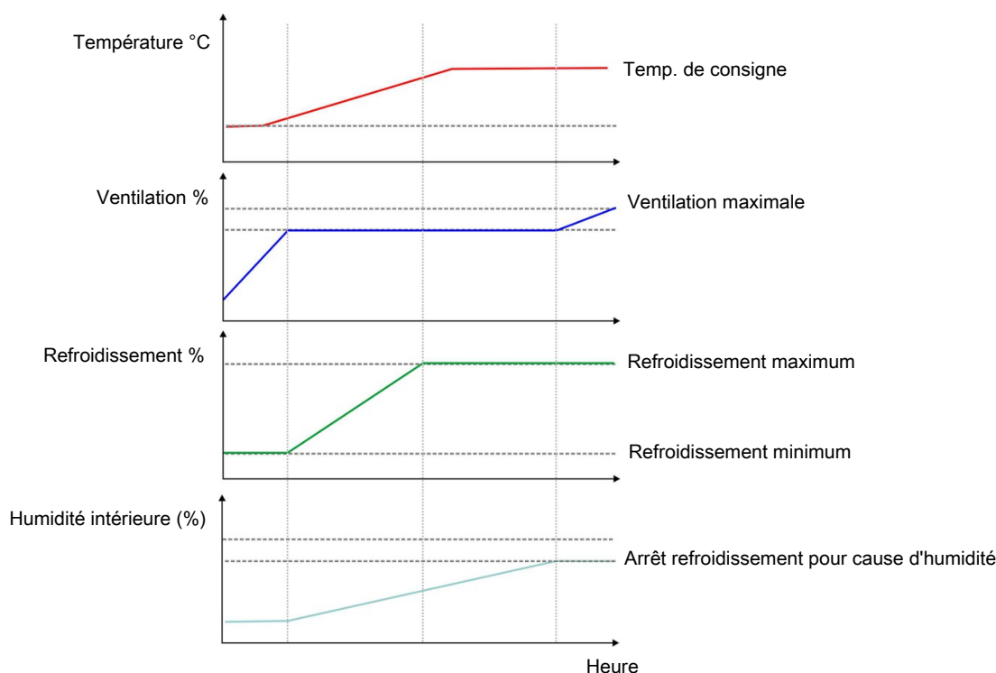
Figure 25: Pour maintenir la température intérieure requise, le refroidissement démarre avant que le niveau de ventilation n'ait atteint la ventilation maximale. Lorsque le refroidissement ne peut plus maintenir la température, la ventilation est augmentée à nouveau.
