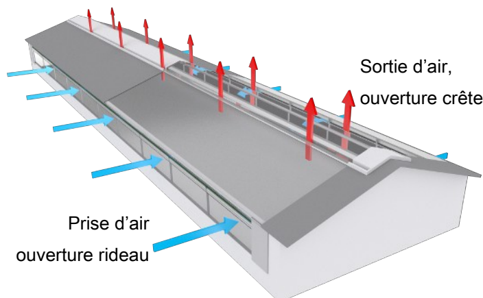
Figure 17: Par exemple, dans un bâtiment à la ventilation naturelle pure avec des ouvertures rideaux sur les côtés du bâtiment et une ouverture crête sur le toit.
