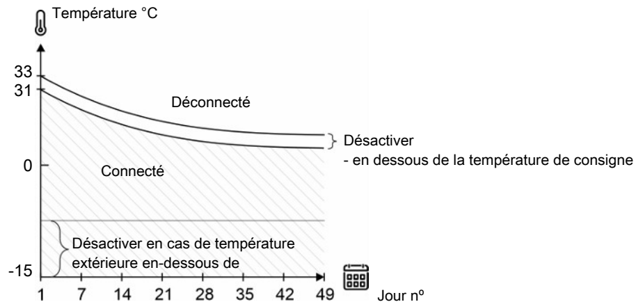
Figure 15: Unité de récupération de chaleur – Limites de température extérieure haute et basse
