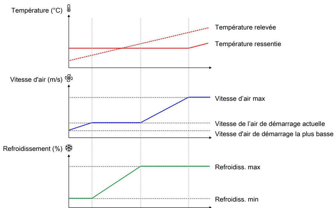
Figure 32: Le refroidissement démarre déjà à une vitesse d'air basse afin de maintenir la température intérieure requise. Lorsque le refroidissement ne parvient pas à maintenir la température, la vitesse d'air est de nouveau augmentée.
